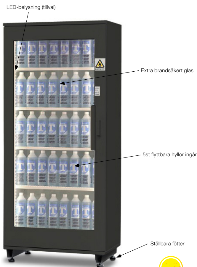
Brandavskiljande skåp NORD460
